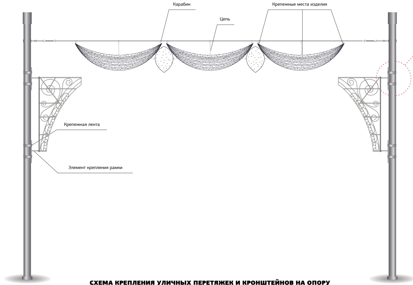
СХЕМА КРЕПЛЕНИЯ УЛИЧНЫХ ПЕРЕТЯЖЕК И КРОНШТЕЙНОВ НА ОПОРУ
